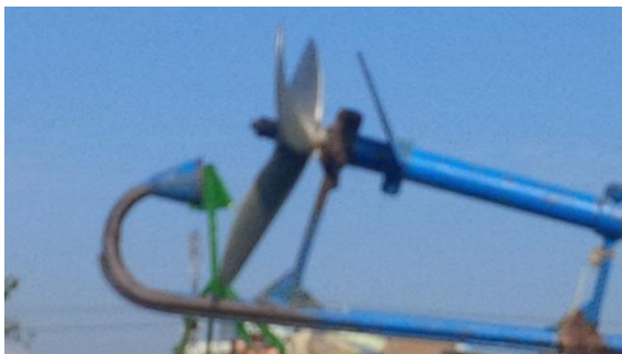
Moteur de bateau à hélice, à refroidissement à eau (voir "l'entonnoir" par lequel l'eau est aspirée par une pompe pour refroidir le moteur)
